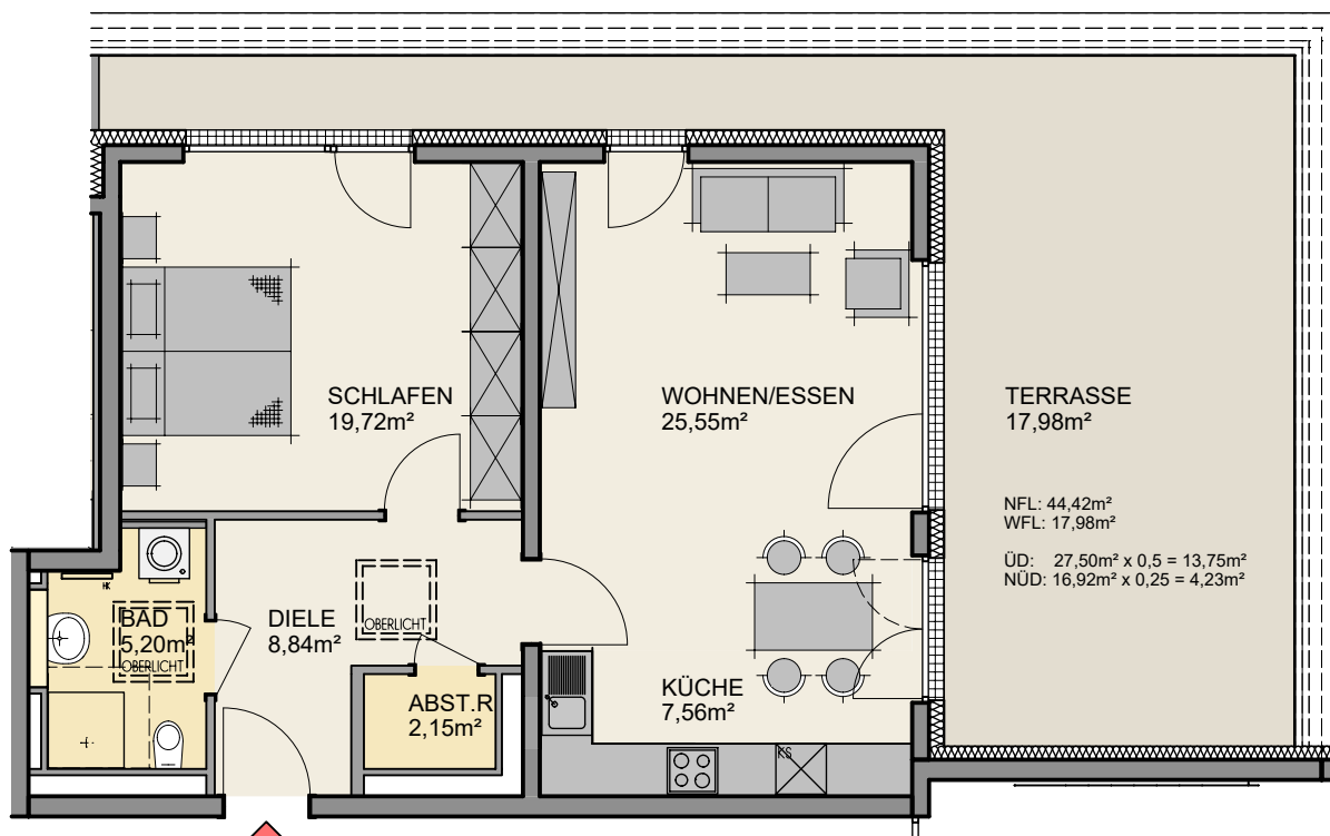
Grundriss 1 : 100
